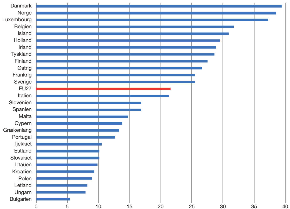
Figur 1. Gennemsnitlig timeløn i udvalgte lande og EU27. 2020. Euro.
